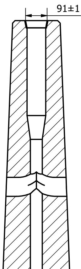
A-A ( 1 : 10 )
