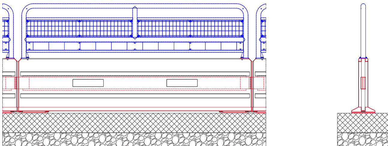
Bild 2 | Detalj från installationsritningen K1002259.
